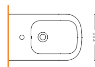
BIDET FILO MURO 56Q BACK TO WALL BIDET 56Q SMMX.S30.F03
