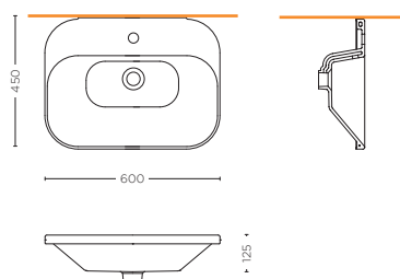
LAVABO DA INCASSO 60 cm COUNTERTOP WASHBASIN 60 cm SMMX.S11.20
