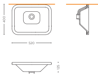
LAVABO DA INCASSO 52 cm COUNTERTOP WASHBASIN 52 cm SMMX.S11.21
