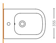
BIDET SOSPESO 50Q WALL HUNG BIDET 50Q SMMX.S30.W01
