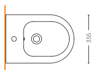
BIDET FILO MURO 50R BACK TO WALL BIDET 50R SMMX.S30.F02
