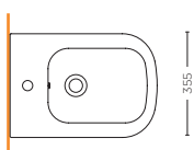
BIDET FILO MURO 50Q BACK TO WALL BIDET 50Q SMMX.S30.F01
