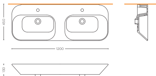
LAVABO 120 cm WASHBASIN 120 cm SMMX.S10.10
