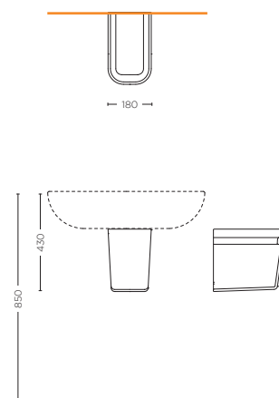
SEMICOLONNA HALF PEDESTAL SMMX.S19.H01
