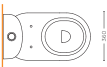
VASO MONOBLOCCO CON CASSETTA SCARICO A PARETE CLOSE COUPLED WC WITH CISTERN P-TRAP SECO.S20.CP01 / SECO.S28.01
