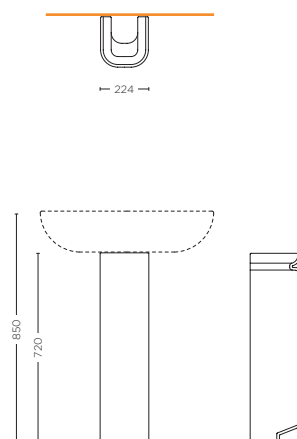
COLONNA PEDESTAL SMMX.S19.F01
