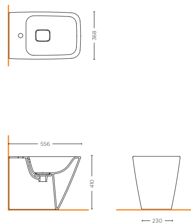
BIDET FILO MURO BACK TO WALL BIDET SCLB.S30.F01
